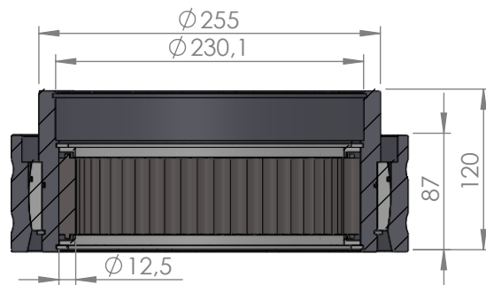
SECTION A-A SCALE 1 : 5
