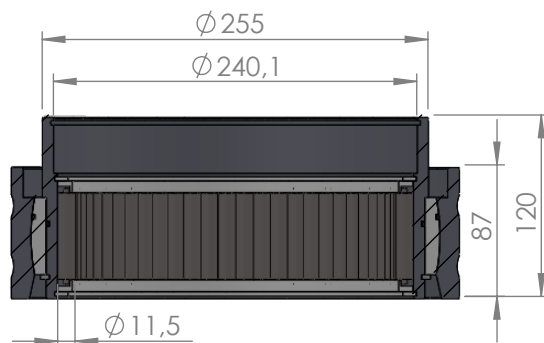
SECTION A-A SCALE 1 : 5
