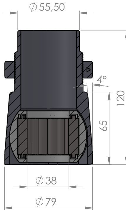
SECTION A-A SCALE 1 : 2
