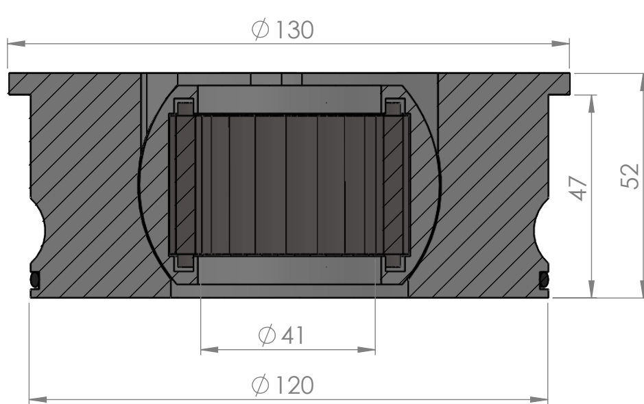
SECTION A-A SCALE 1 : 1.2
