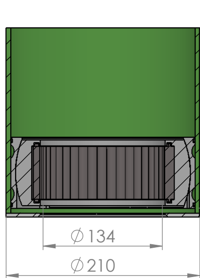
SECTION A-A SCALE 1 : 4
