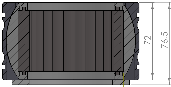
SECTION A-A SCALE 1 : 1.75
