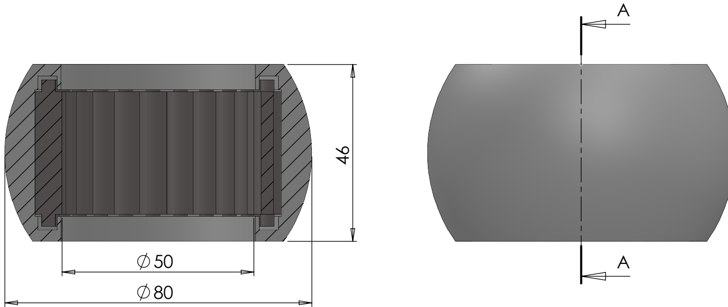
SECTION A-A SCALE 1 : 1
