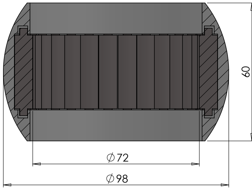
SECTION A-A
