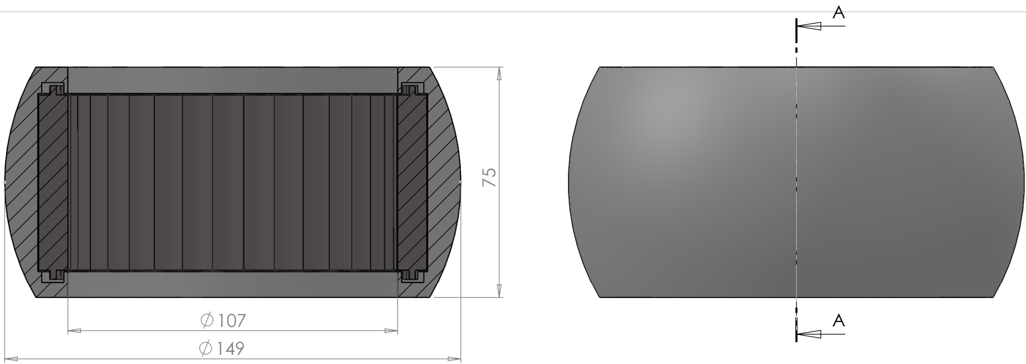
SECTION A-A SCALE 1 : 1.25
