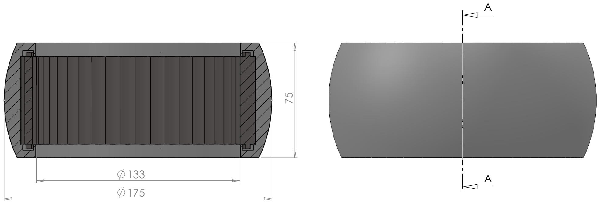
SECTION A-A SCALE 1 : 1.5
