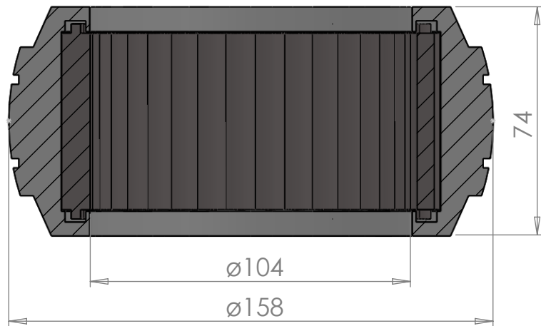
SECTION A-A SCALE 1 : 1.75
